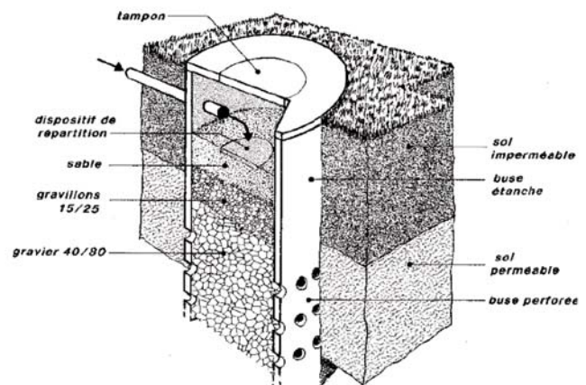
Schéma de principe du rejet des eaux traitées par puits d'infiltration
